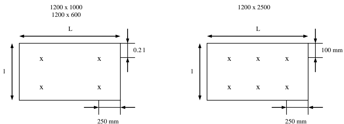
Fig. 1: Schéma de pose des fixations dans le cas de panneaux fixés mécaniquement
