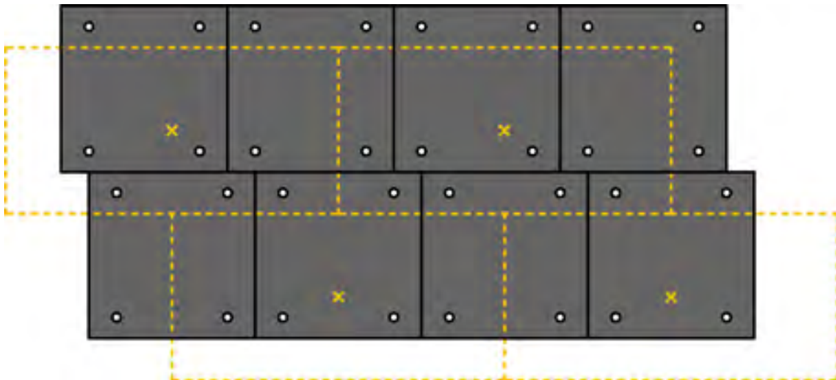
Eristelevyjen kiinnitys ja limitys
