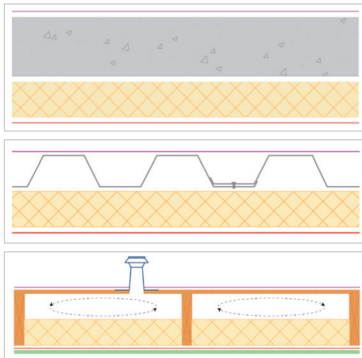
Afbeelding 6: Koud dak - NIET toegestaan!
