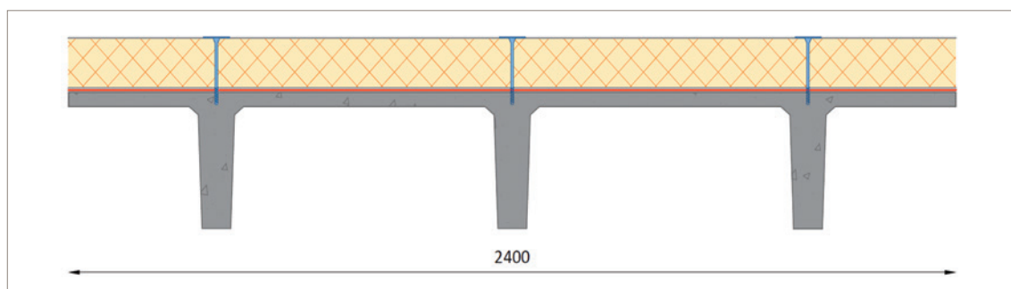
Afbeelding 19: Voorbeeld van dubbele TT-ligger met bevestiging in de 'T'-ribben
