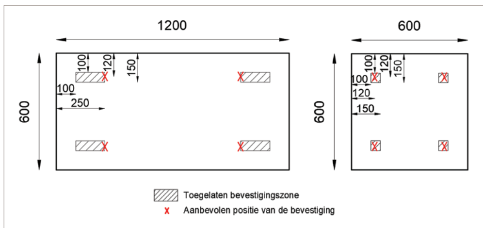
Afbeelding 17: Bevestigingspatroon - Kleine platen
