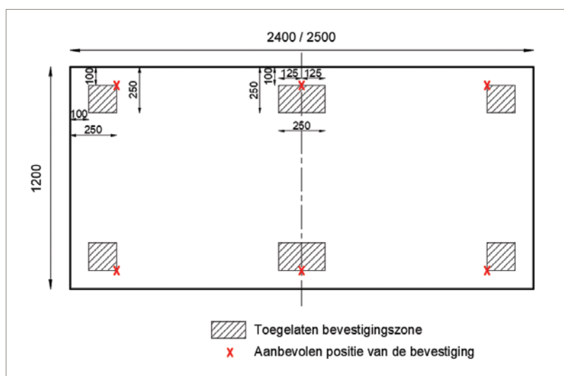
Afbeelding 15: Bevestigingspatroon - Grote platen
