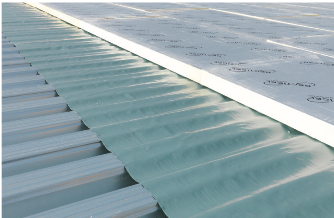
Afbeelding 24: Plaatsing van isolatieplaten op een stalen ondergrond
