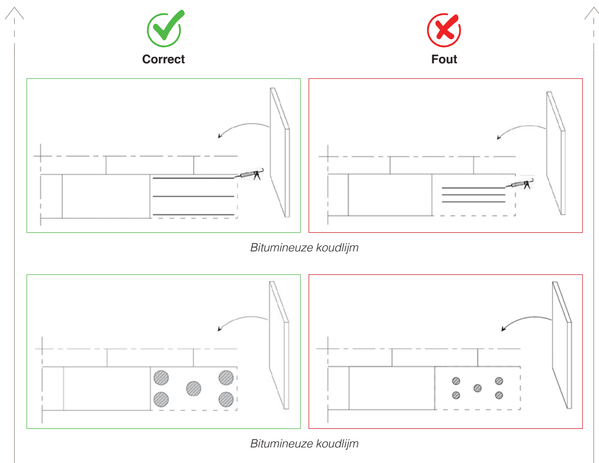
Afbeelding 30: Verlijmde opbouw - Lijmpatroon (principetekeningen)
