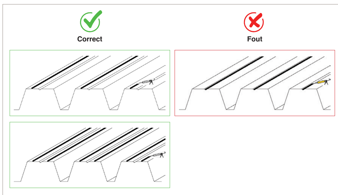
Afbeelding 31: Rechtstreeks op steeldeck lijmen (principetekeningen)
