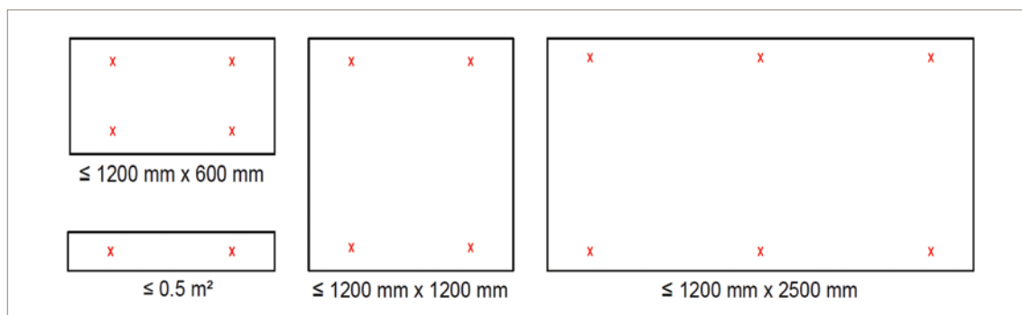
Afbeelding 18: Minimaal aantal bevestigingen voor verzaagde stukken
