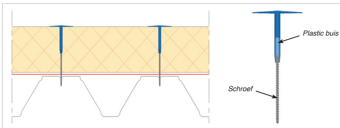
Afbeelding 28: Thermisch verbeterd bevestigingssysteem
