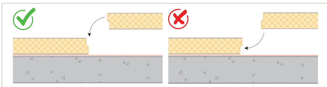
Afbeelding 29: Installatie van isolatieplaten met sponning (links: correcte toepassing, rechts: foutieve toepassing)
