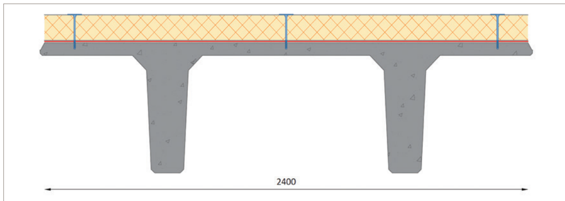
Afbeelding 20: Voorbeeld van enkelvoudige TT-ligger met bevestiging in de ondergrond
