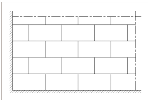
Afbeelding 11: Geschrante voegen in het geval van een opbouw met één isolatielaag
