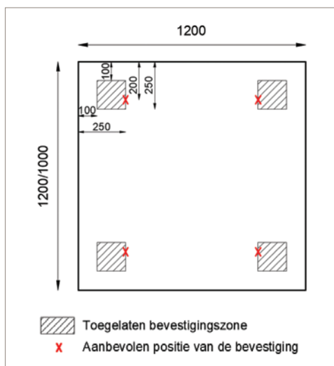
Afbeelding 16: Bevestigingspatroon - Middelgrote platen
