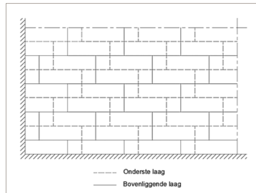
Afbeelding 12: Geschrante voegen in het geval van een opbouw met meerdere lagen
