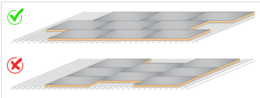
Afbeelding 23: Plaatsing van isolatieplaten op een stalen ondergrond (Boven: correct patroon - Onder: fout patroon)
