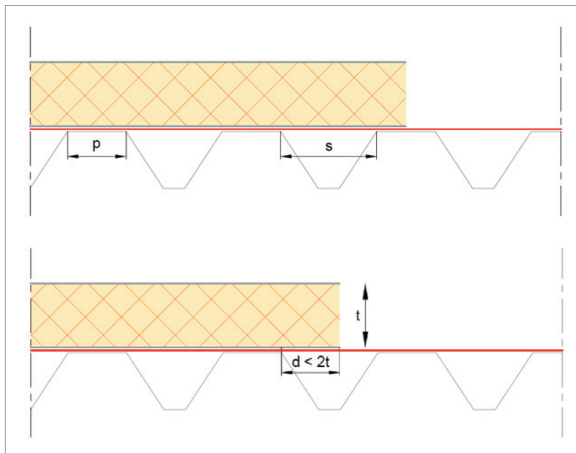
Afbeelding 22: Plaatsing van isolatieplaten op een stalen ondergrond (Boven: geprefereerde installatie - ondersteunde randen; Onder: Beperking van uitkraging voor t \geq 50 mm)
