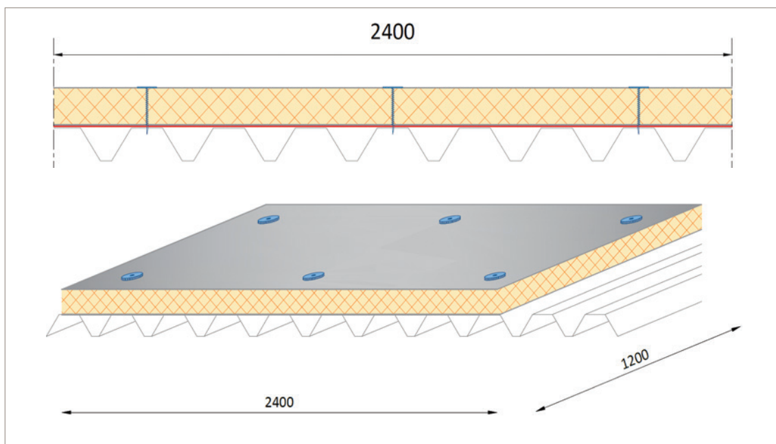
Afbeelding 21: Bevestiging van isolatieplaten op een stalen ondergrond (19)
