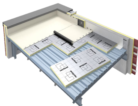
Exemple de pose directe sur bac acier
