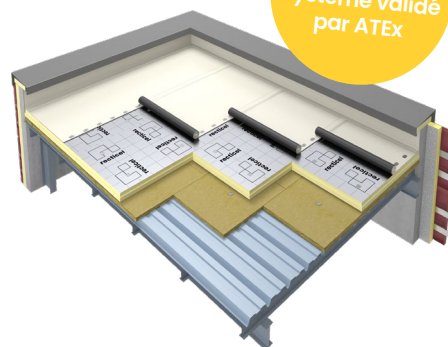
Exemple de pose avec écran thermique
