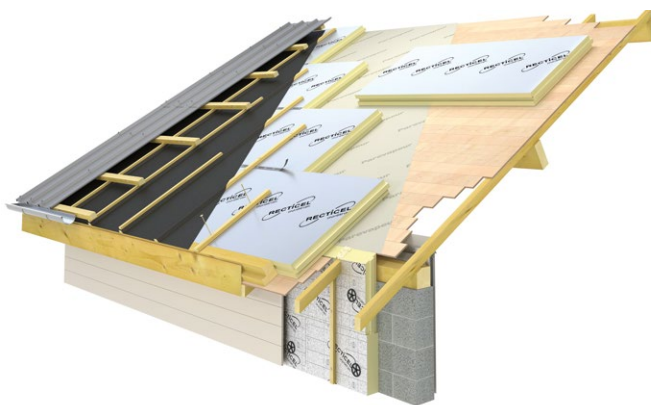
Pose sur support rigide continu avec pare-vapeur et étanchéité obligatoire
