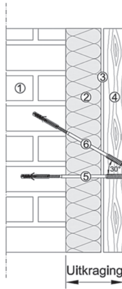
Verticale doorsnede
